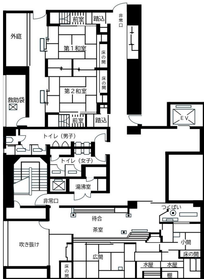
和室・茶室配置図
